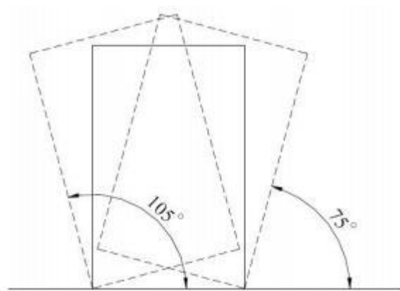
图2.1.2 搬运倾角
