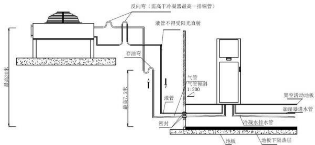
图 2.3.2 冷凝器高于压缩机的安装示意图
